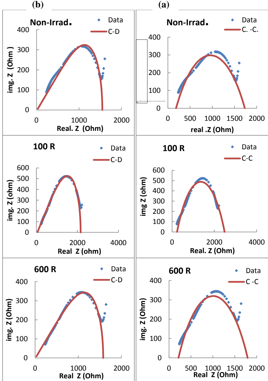
شكل 3. موائمة نموذج كول (C-C) في العمود (a) ونموذج كول- دافيدسون (C-D) في العمود (b) لبيانات المعاوقة الكهربائية المركبة لأنسجة غير مشععة في الصف الاول ومشععة بـ 100 راد في الصف الثاني ومشععة 600 راد بالصف الأخير.
