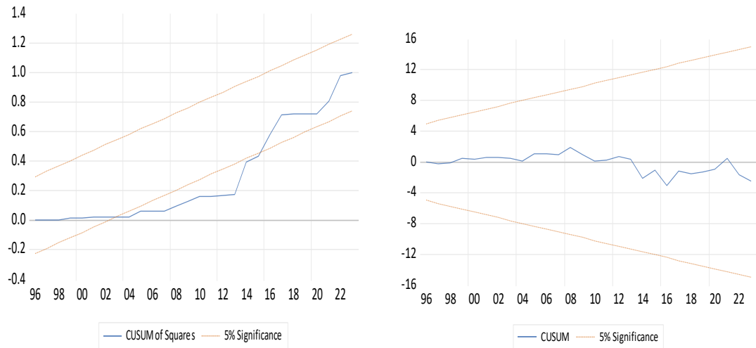
شكل رقم (5) اختبار الاستقرار الهيكلي لنموذج ARDL المقدر
