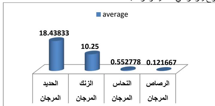
شكل 4. متوسطات تركيزات المعادن الثقيلة في سمك المرجان.
