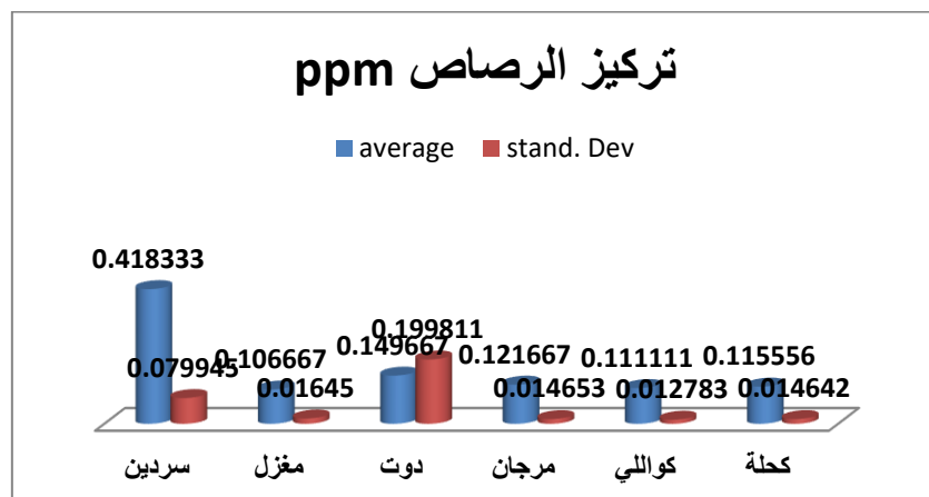
شكل 10. المتوسط الحسابي والانحراف المعياري لمعدن الرصاص في الاسماك المدروسة
