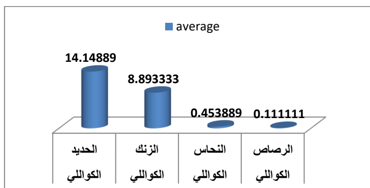
شكل 5. متوسطات تركيزات المعادن الثقيلة في سمك الكواللي.
