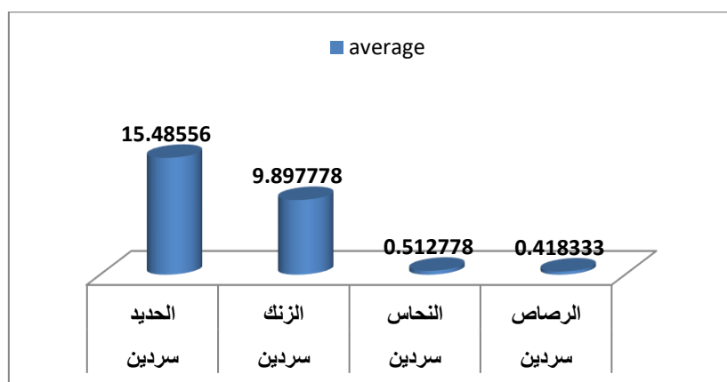
شكل 1. متوسطات تراكيز المعادن الثقيلة في سمك السردين.
