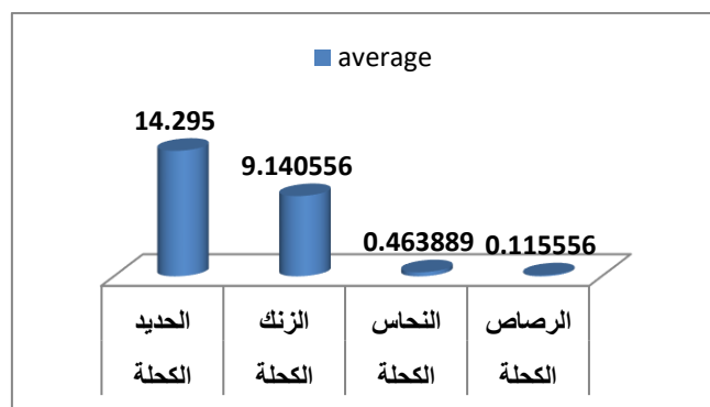
شكل 6. متوسطات تركيزات المعادن الثقيلة في سمك الكحلة.
