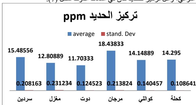
شكل 7. المتوسط الحسابي والانحراف المعياري لمعدن الحديد في الأسماك المدروسة.
