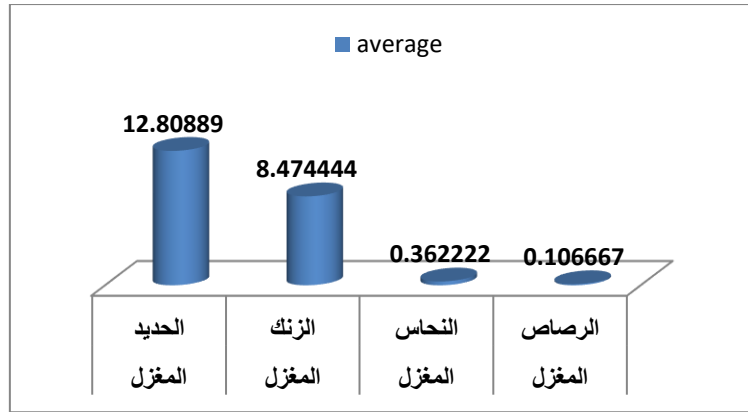
شكل 2. متوسطات تركيزات المعادن الثقيلة في سمك المغزل.
