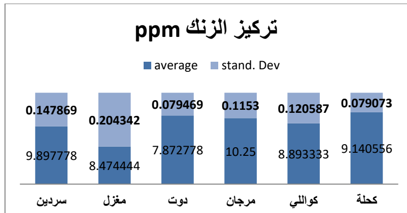
شكل 8. المتوسط الحسابي والانحراف المعياري لمعدن الزنك في الاسماك المدروسة.
