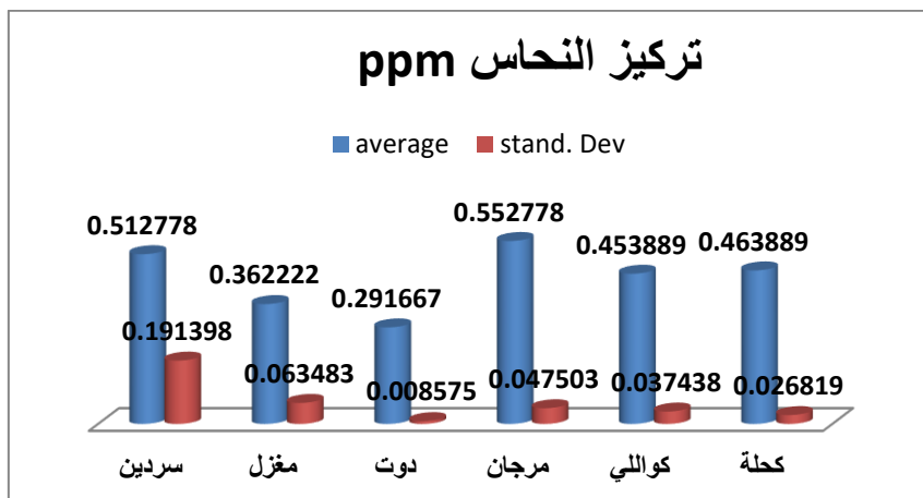
شكل 9. المتوسط الحسابي والانحراف المعياري لمعدن النحاس في الاسماك المدروسة
