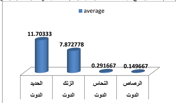
شكل 3. متوسطات تركيزات المعادن الثقيلة في سمك الدوث.
