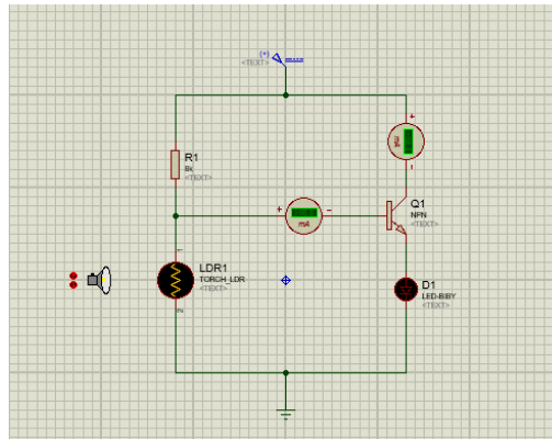
شكل (9) تصميم دائرة الاضاءة الليلية في بروتس
