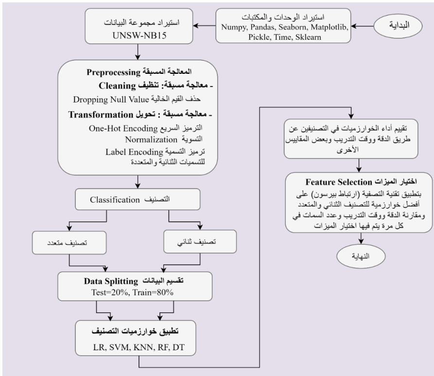
شكل (2) المخطط الانسيابي المتبع في هذا البحث [22].
