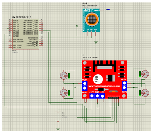
شكل (2) النظام المصمم من خلال بروتوس
