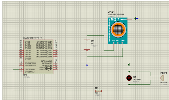
شكل (6) دائرة اختبار حساس الغاز
