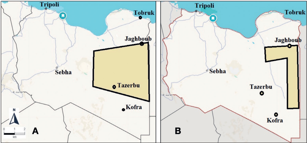
Figure 1. Study areas surveyed for Sooty Falcon nests: 2024 (A) and 2020–2023 (B) 1. ábra A hamvas sólyom fészkek keresése során felmért mintaterületek: 2024 (A) és 2020–2023 (B)
