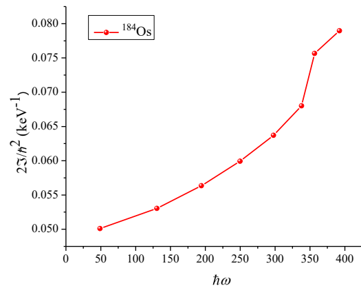
الشكل 5. عزم القصور الذاتي دالة للطاقة الدورانية لنظائر ^{178-184}\text{Os}
