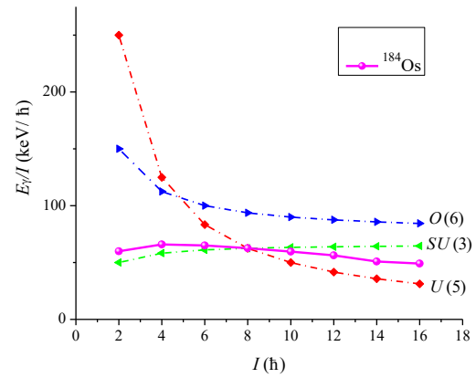
الشكل 4. منحنيات E-GOS للنظائر ^{178-184}\text{Os} مقارنة مع المنحنيات
