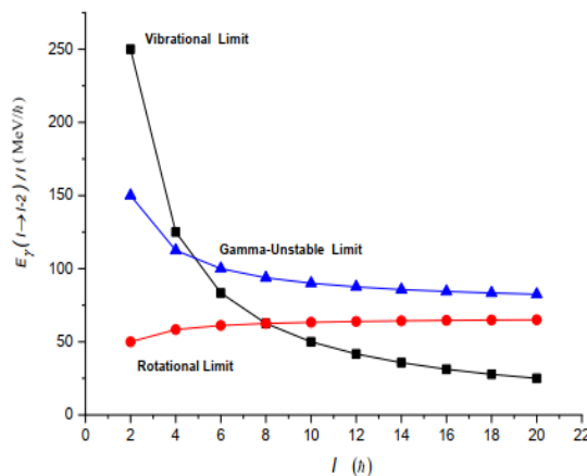
الشكل 1. منحنيات E-GOS للتحديدات الثلاثة الاهتزازية وجاما الناعمة والدورانية [14]
