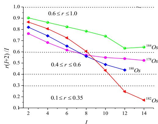
الشكل 3. النسبة r(I+2/I) كدالة في الزخم الزاوي لنظائر
