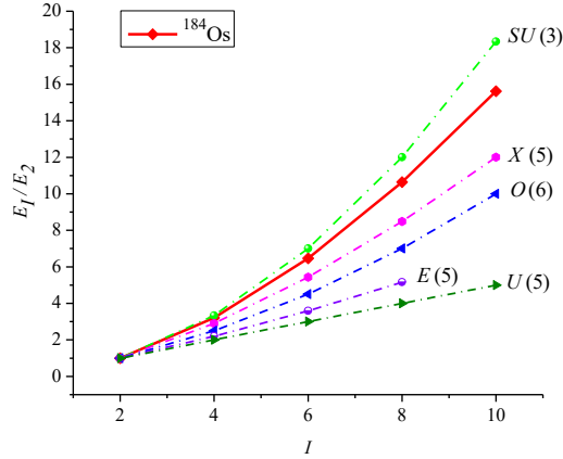
الشكل 2. قيم نسب الطاقة E(I_1^+)/E(2_1^+) النموذجية لكل تحديد وقيم النسب التجريبية [20] للنظائر ^{178-184}\text{Os}
